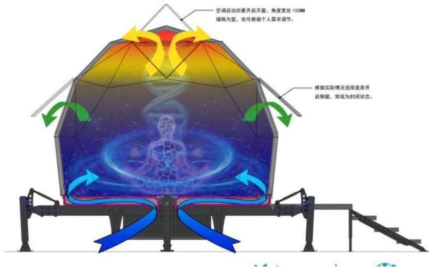
潮汐制冷示意
